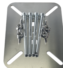
Art. nr. 720308 •79443449 X 4stk •7930001 X 4stk
