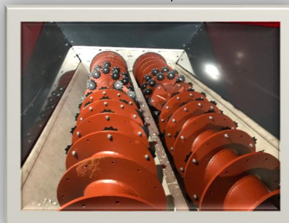
Horisontale skruer med 100 kniver
