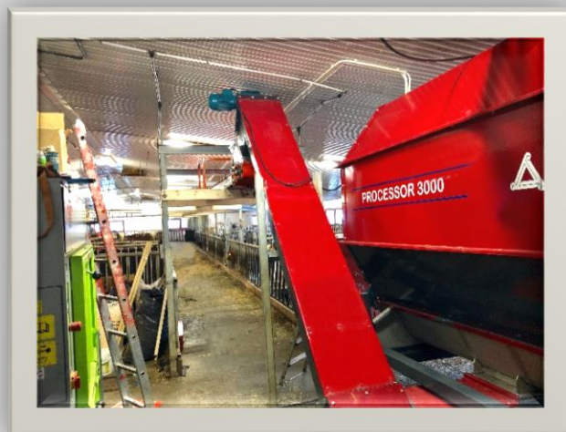
Skruer tar her fôret opp på utfôringsband
