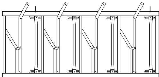
Ungdyr: Fanggitter med indstillelig halsrør.
