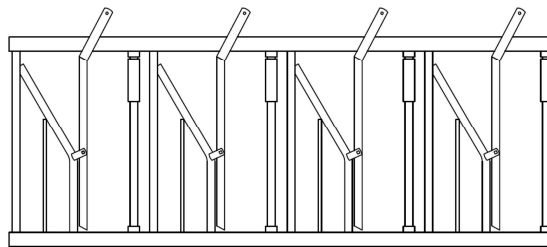
Ko og Kødkvæg: fanggitter med fjederrør
